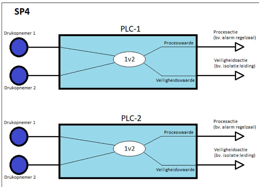
Figuur 7-3 Schematische werking van de procesregeling en veiligheidsregeling in SP4
