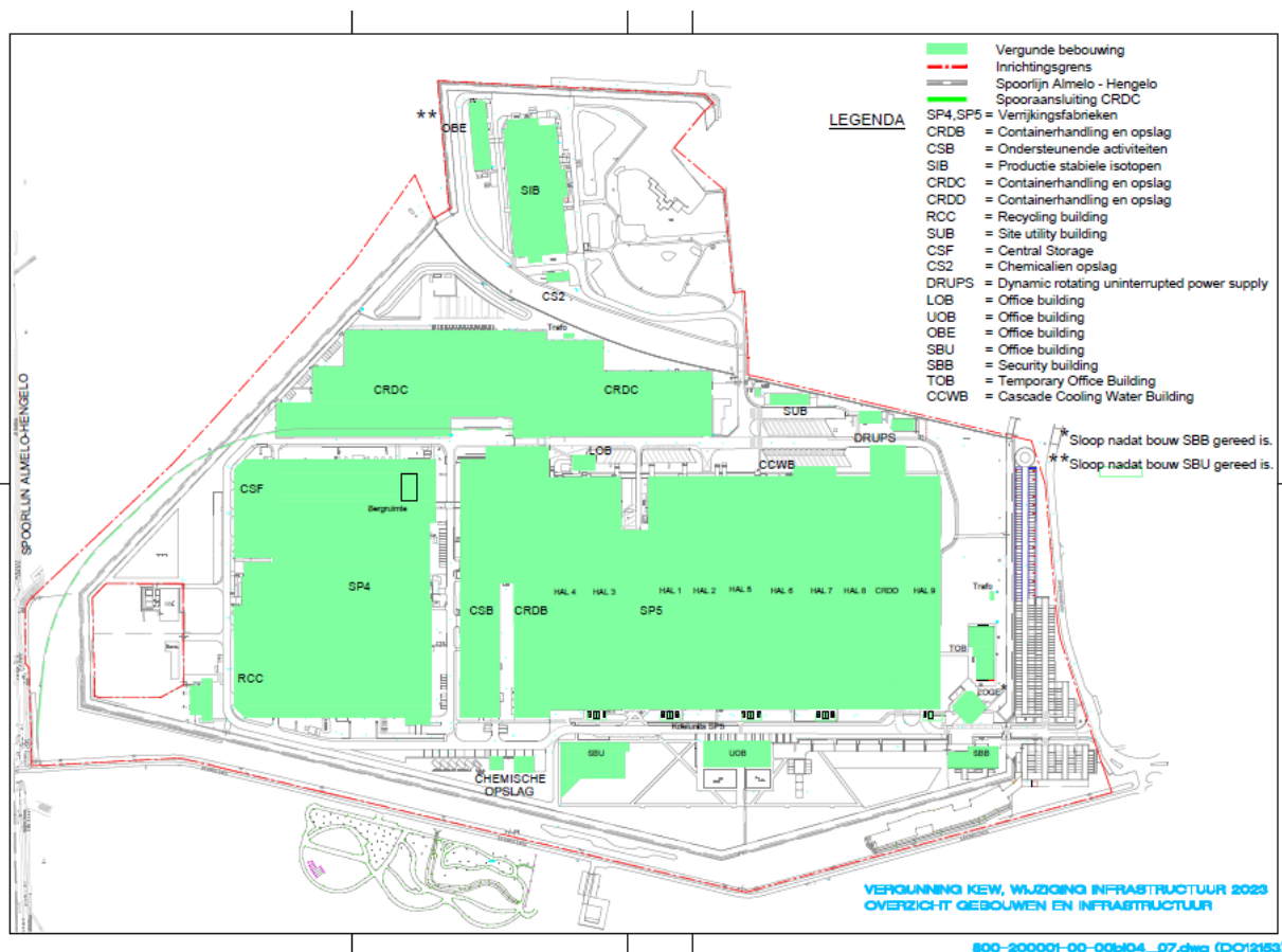
Figuur 1-2 Plattegrond Urenco site met terreingrens en overzicht en locatie van de gebouwen
