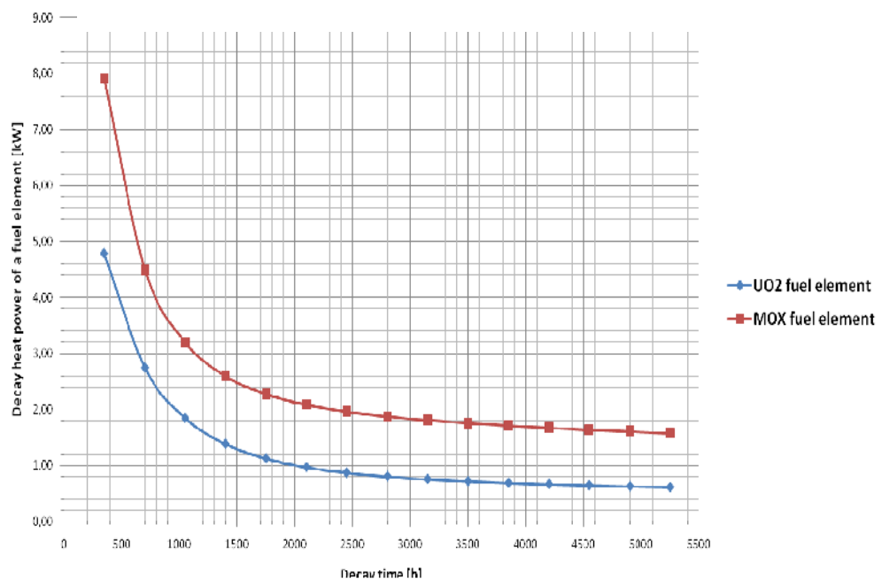
Fig. 4.1 Vervalwarmte (kW) van resp. een enkel splijstofelement UO 2 en MOX als functie van de tijd (350uur < t < 5200 uur)
