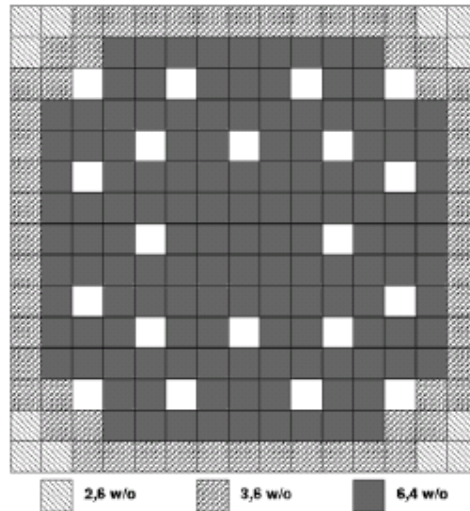
Schema van de positie van verschillende MOX splijtstofstaven in een MOX element. De blanco vakken betreffen regelstafposities.
