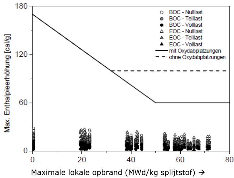
Fig. 7.6 Maximale te bereiken enthalpiesprong als functie van de opbrand
