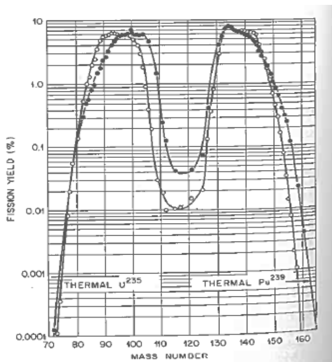
Fig. 12.1 Splijtingsopbrengst Pu-239 en U-235
