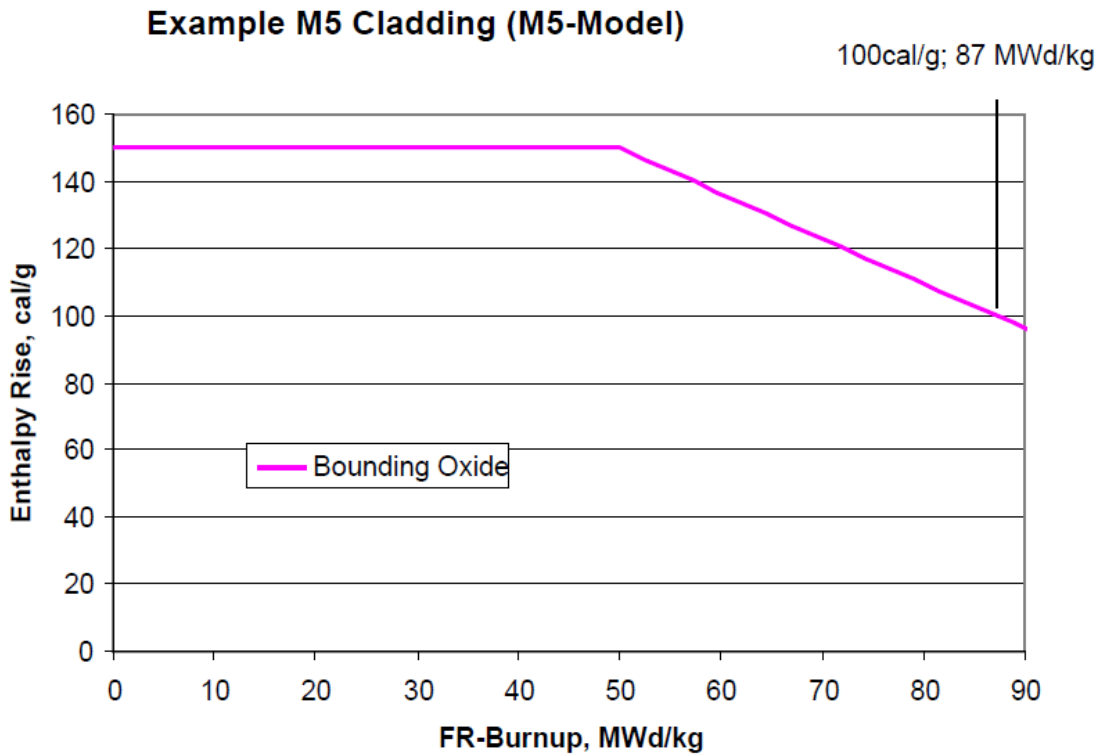
Fig. 7.8 Veiligheidscriteria VS m.b.t. regelstaafuitworp ongevallen voor M5 splijstofomhulling materiaal.
