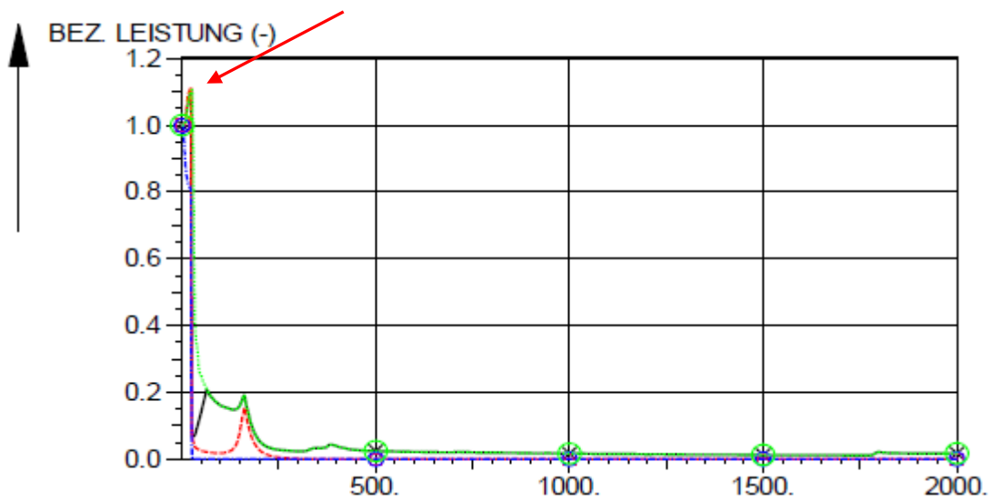
Fig. 7.4 Reaktiviteit en vermogen reactor met MOX-kern t.g.v. "Onbedoeld openen van de turbine omloopkleppen"; vermogensbegrenzing grijpt niet in; reactor scamt bij 110% vermogen.
