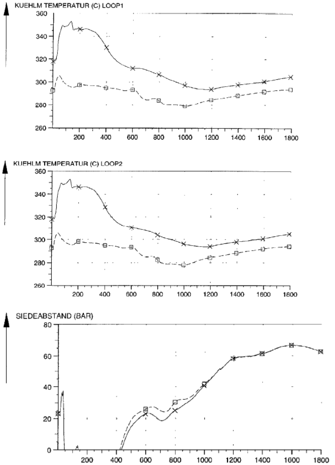
Fig. 7.13 Temperatuur primaire koelmiddel (°C) en kookafstand (bar) gedurende ATWS. Tijd is in seconden
