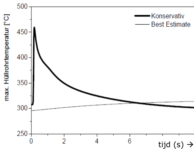
Fig. 7.5 Maximale temperatuur splijstofomhulling (MOX)
