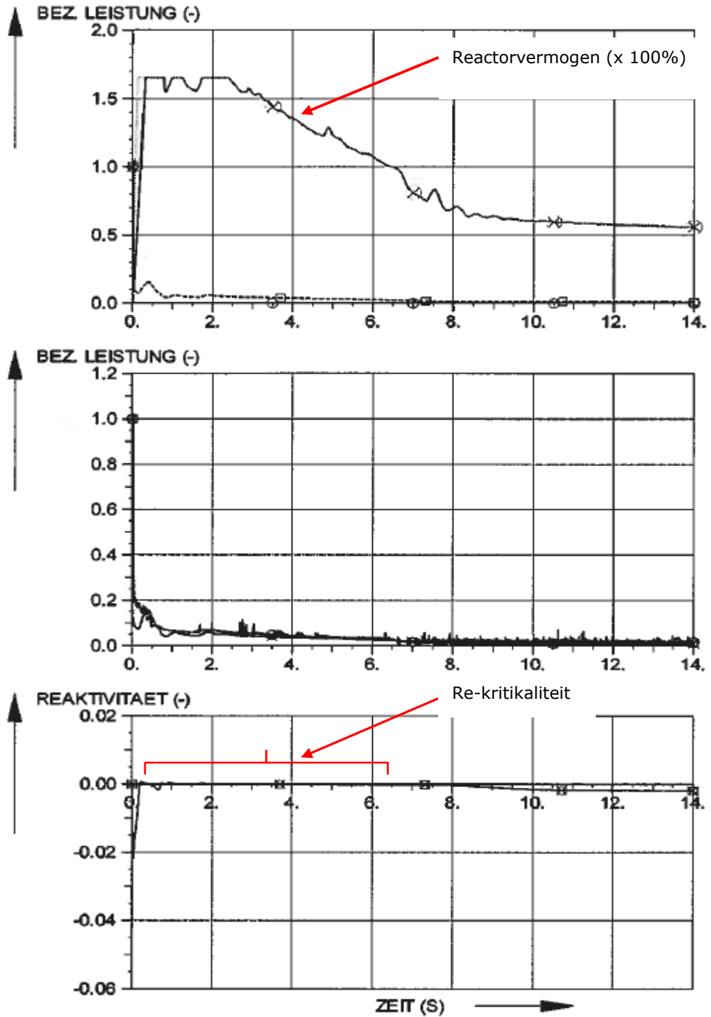
Fig. 7.1 Re-kritikaliteit MOX-kern bij breuk hoofdstoomleiding t.g.v. aardbeving
