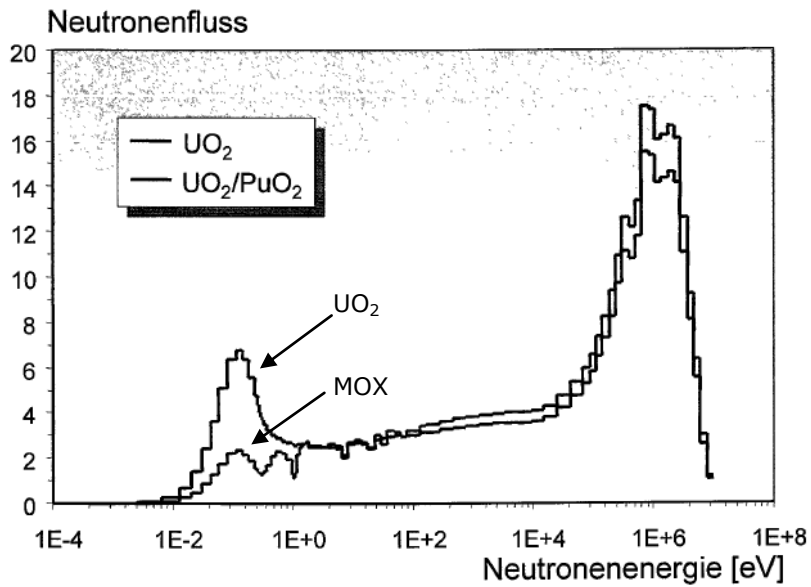
Fig. 4.5 Typische neutronenflux van een MOX-splijstofelement en een \text{UO}_2 splijstofelement
