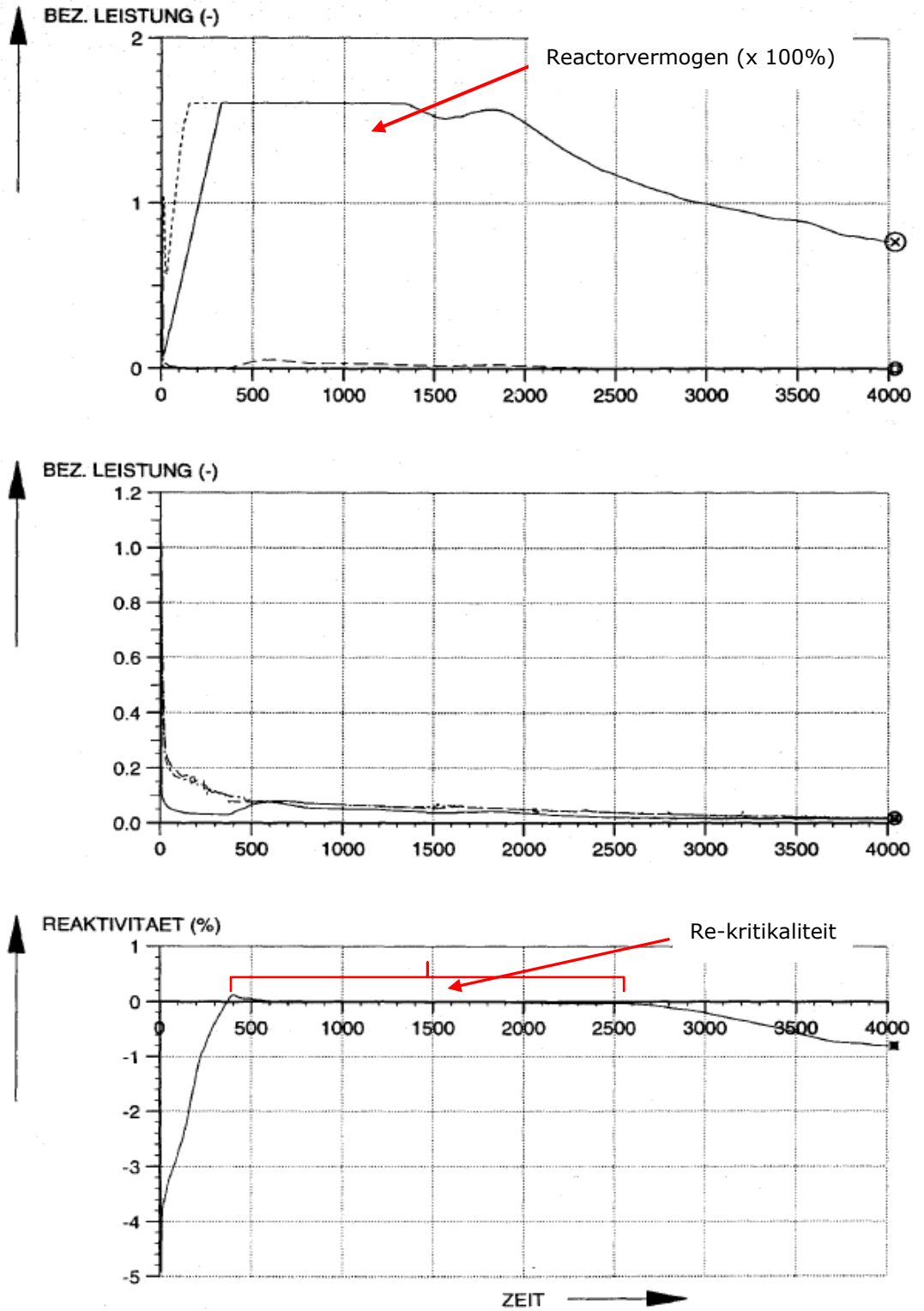
Fig. 7.2 Re-kritikaliteit 4.4% verrijkte UO_2 kern bij hoofdstoomleidingbreuk t.g.v. aardbeving
