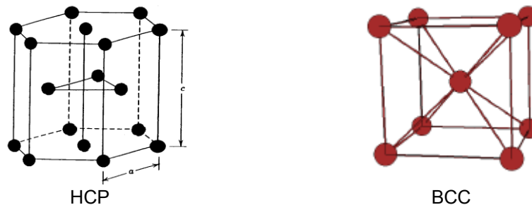
Fig 7.10 Hexagonaal dicht oepengepakt rooster HCP en kubisch ruimtelijk gecentreerd rooster BCC
