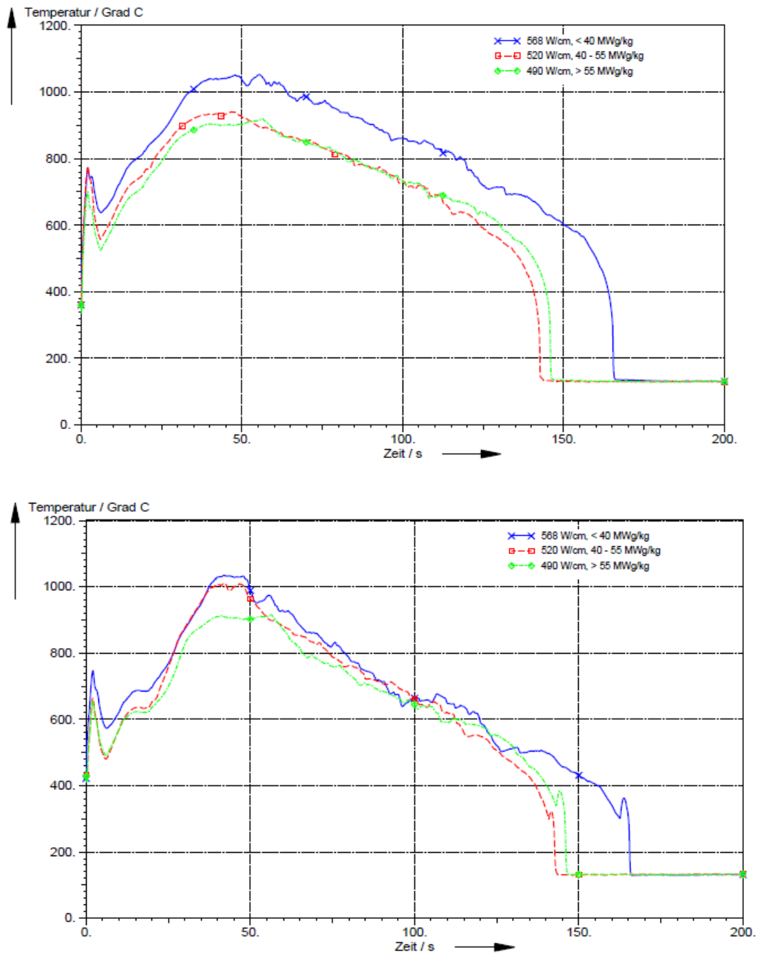
Fig. 7.9 Verloop van de temperatuur van de splijstofomhulling (cladding) bij een groot Koelmiddel Verlies Ongeval; boven zonder opzwellen en barsten van de cladding en onder met opzwellen en barsten van de cladding
